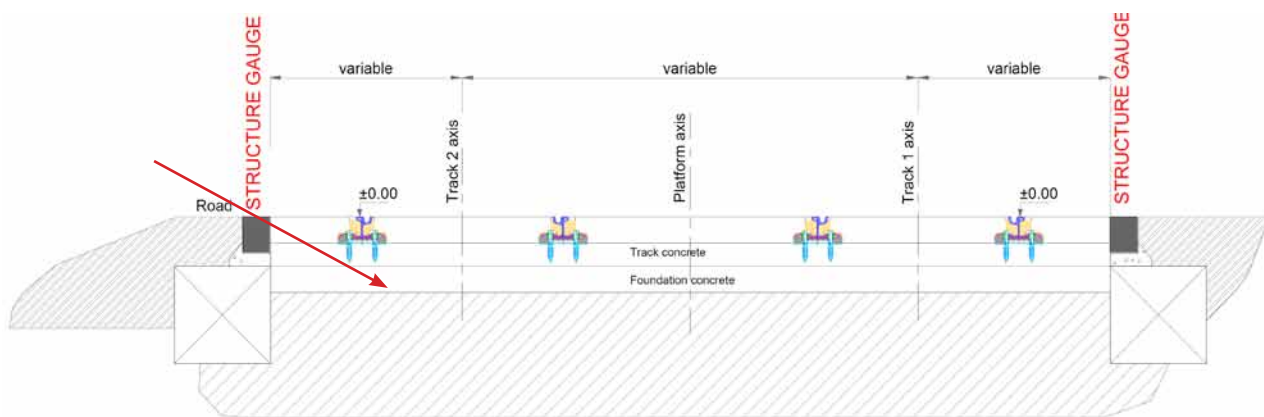
Figur 9-3: Sporkonstruktion med vibrationsdæmpende måtte under betonpladen.
